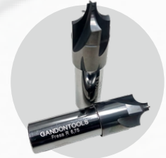
FRESA MD PERFIL ESPECIAL
